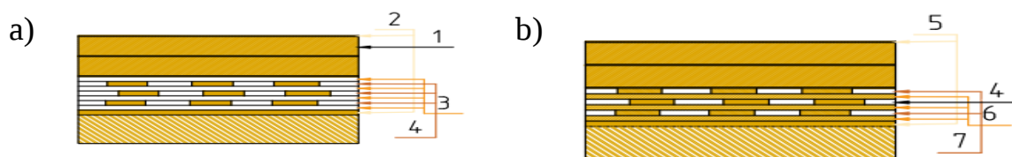
4-rasm. Izolyasiya qilishning variantlari: a) – bitum mastika (BM-1); b) – rulonli izolyasiya (IR); 1 – himoya qatlami; 2 – bitumli gruntovka; 3 – bitumli mastika; 4 – armaturalovchi material; 5 – izolli gruntovka; 6 – rulonli izol; 7 – izolli mastika
