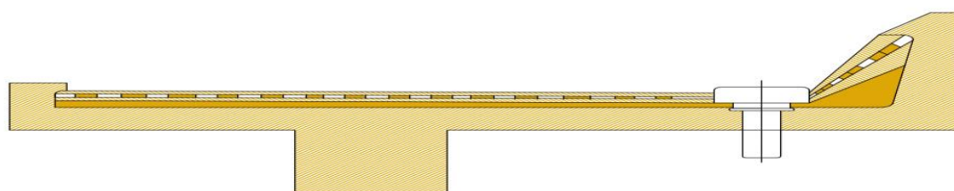
2-rasm. Ballast koritasining gidroizolyasiyasi ko'ndalang kesimi
